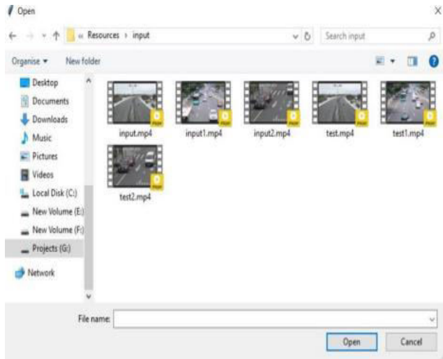
Fig.2. Input video.
