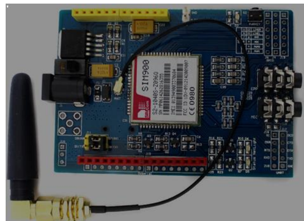
Figure3 - Simcom SIM900 GSM MODULE
